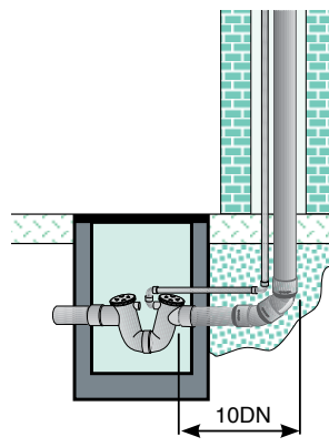
Ventilazione collegata con Sifone A-N
